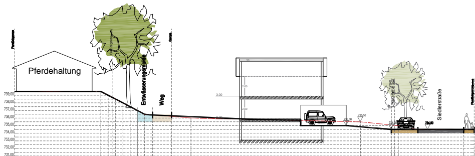
Schnitte AA
