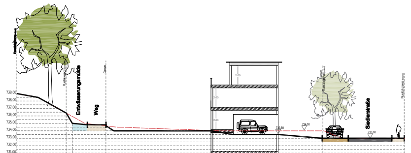
Schnitte BB'
